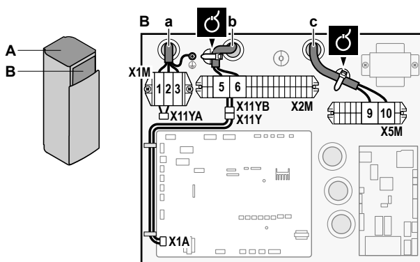
a Prepojovací kábel (=hlavné elektrické napájanie) b Elektrické napájanie s normálnou sadzbou za kWh c Kontakt preferenčného elektrického napájania
