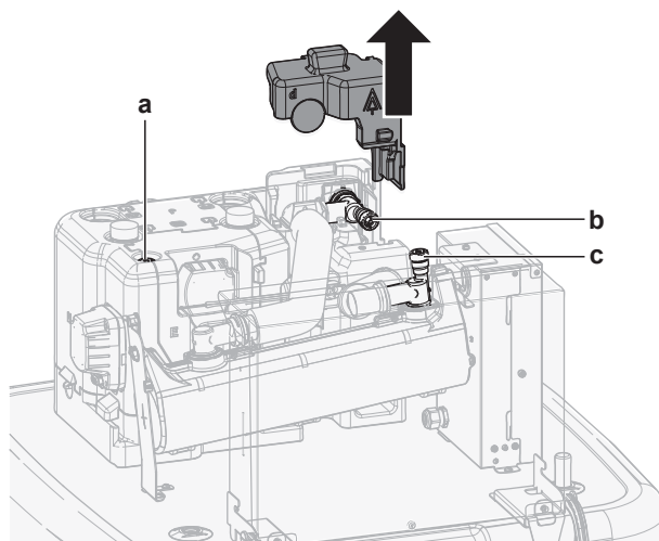
a, b, c Manuálny odvzdušňovací ventil
